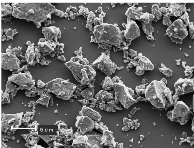
AC ダスト Fine (A2)
